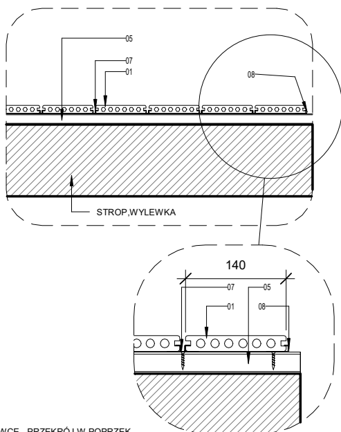
SYSTEM NA WYLEWCE - PRZEKRÓJ W POPRZEK
