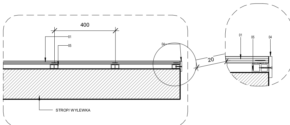
SYSTEM NA WYLEWCE - PRZEKRÓJ W POPRZEK
