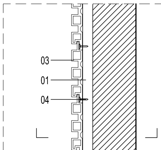
DETAL - RZUT
