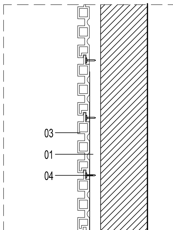
DETAL - PRZEKRÓJ
