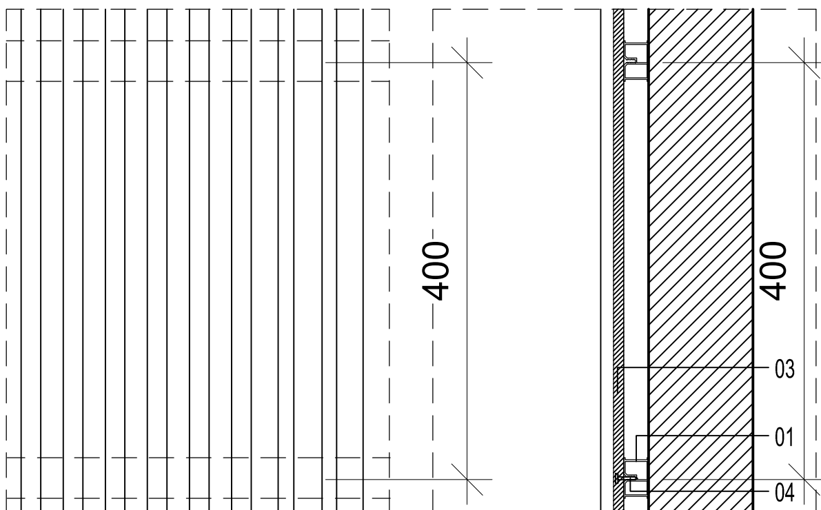
DETAL - ELEWACJA
